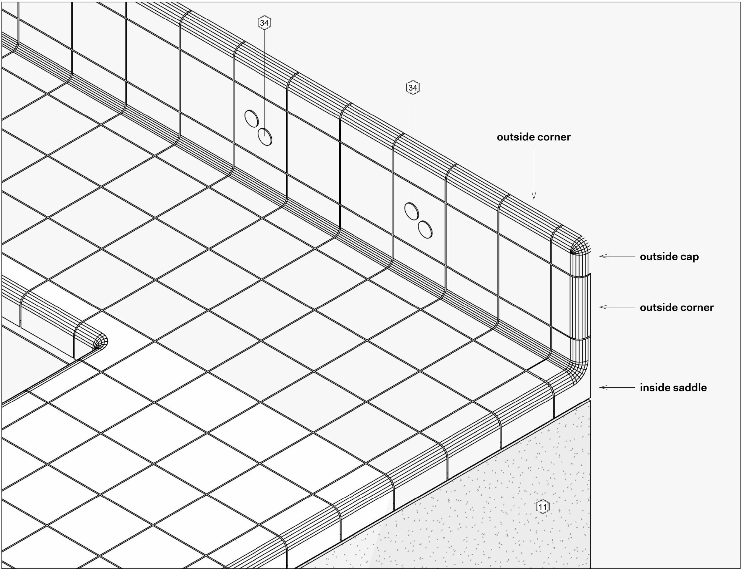
Tile Counter Edge Detail
